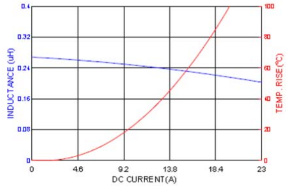
HMPL0502HP-R24
