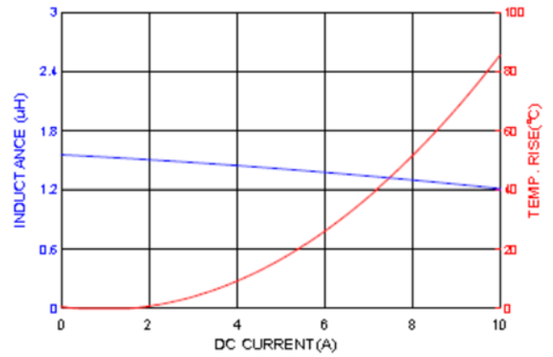
HMPL0502HP-1R5
